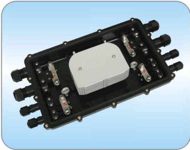
9006型接头盒剖面图
