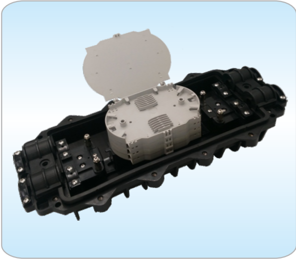
6020型接头盒剖面图
