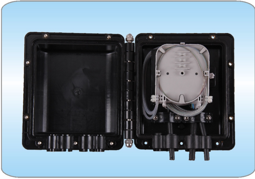
6017型接头盒剖面图（正面）
